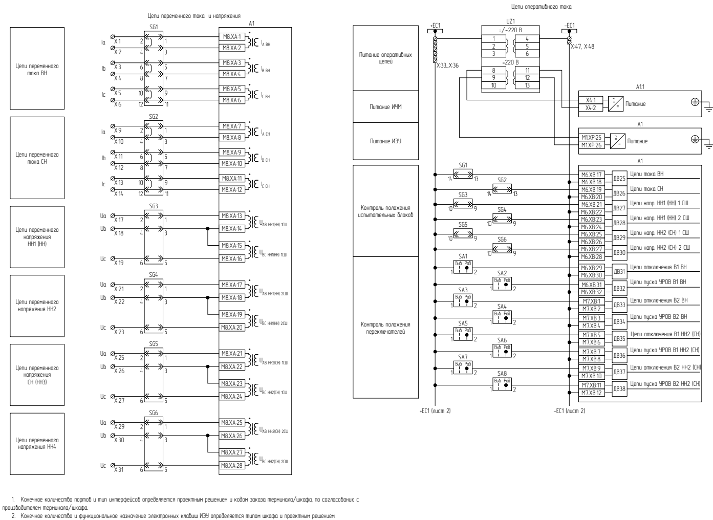
Рисунок В.1 – Схема электрическая принципиальная (часть 1)
